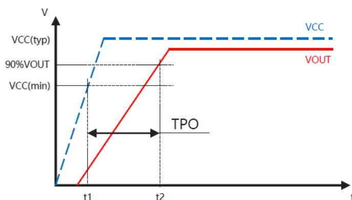
图 1：上电时间定义
